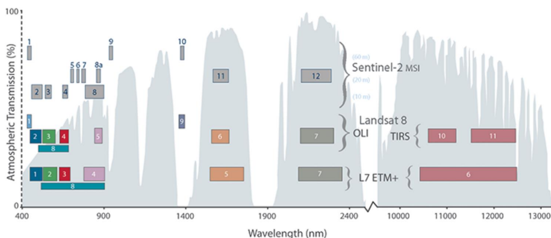
Figura 2 Distribución espectral de bandas.
