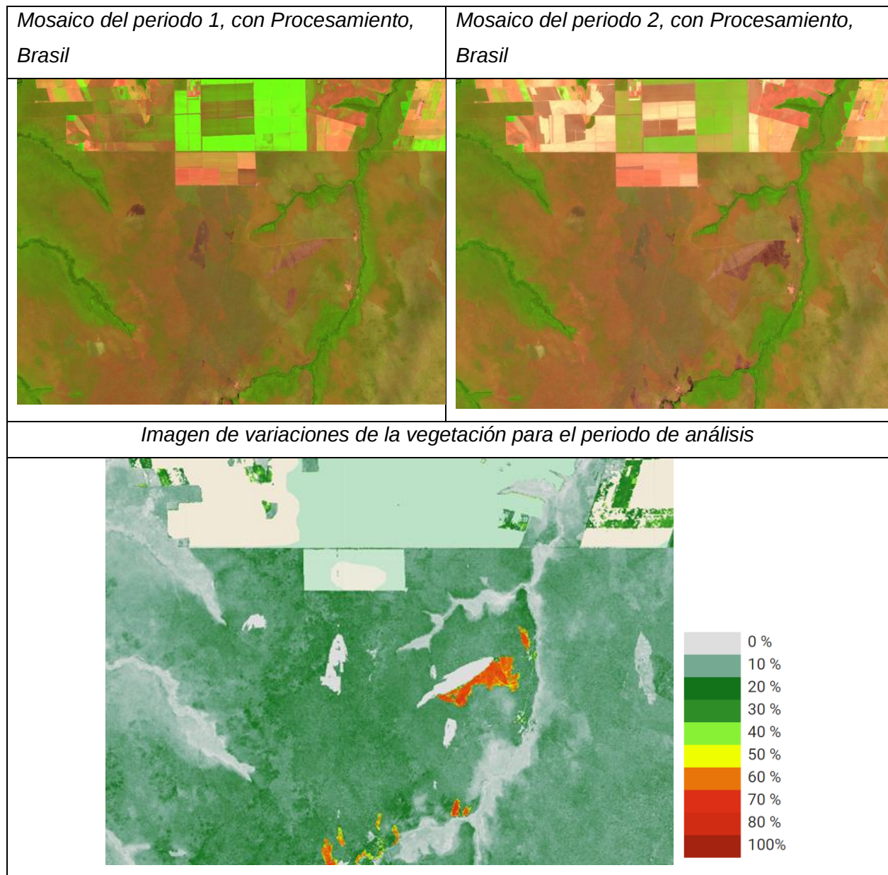
Figura 8 Caso de cicatriz de quema en Brasil
