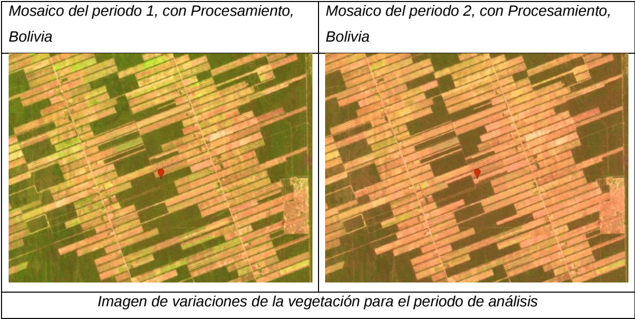
Figura 10 Deforestación en Bolivia
